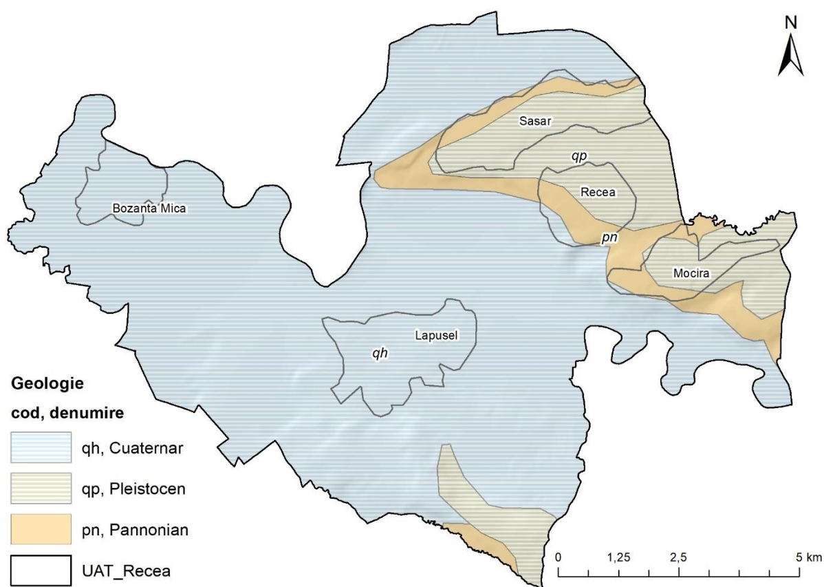
Fig. 2 – Harta petrografică a comunei Recea
