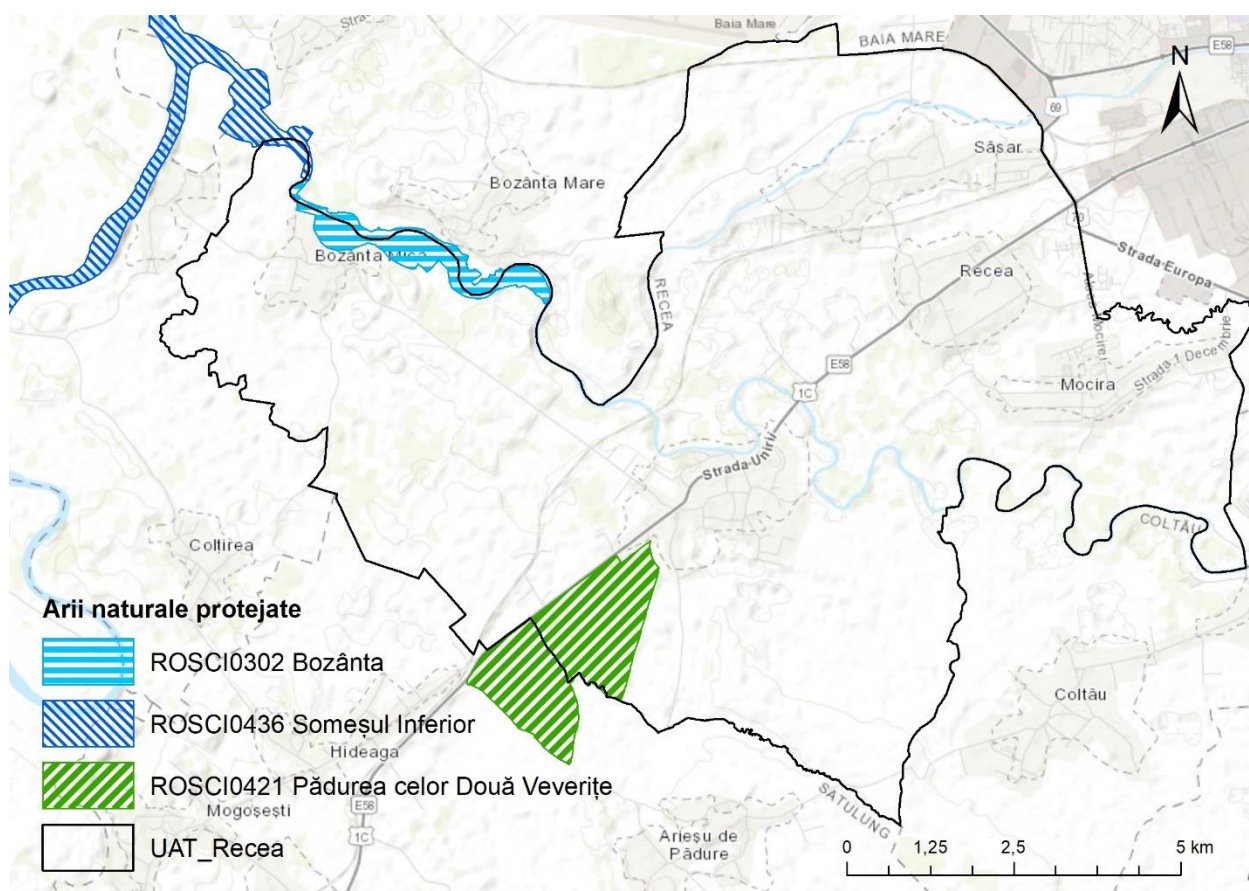
Fig. 10 – Localizarea siturilor Natura 2000 în Comuna Recea
