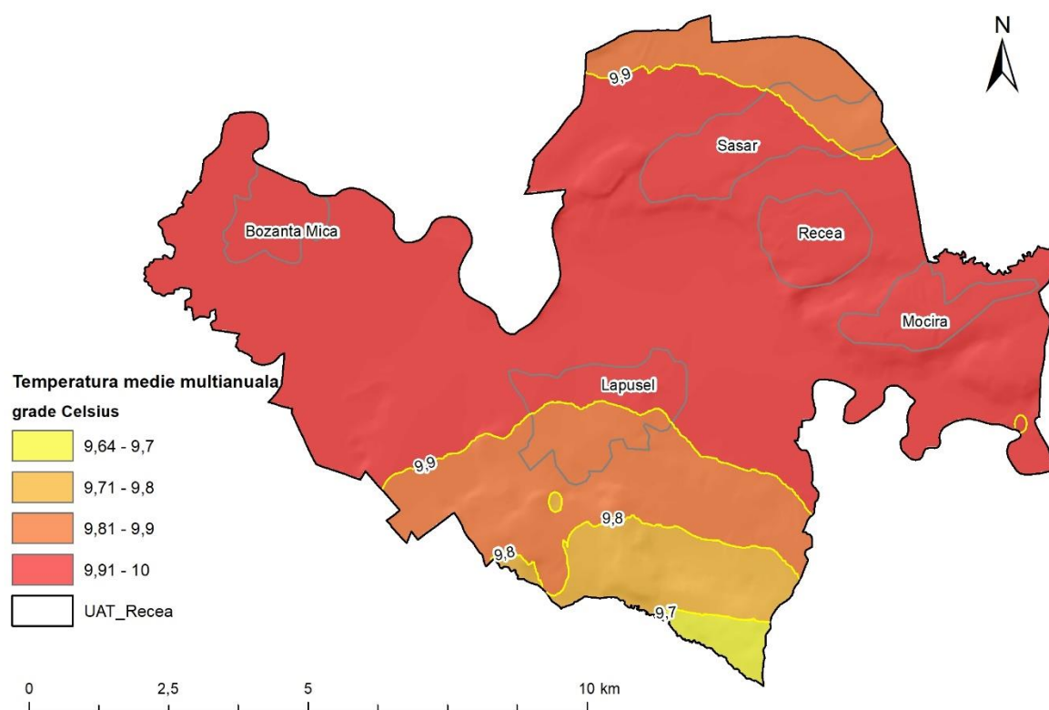
Fig. 4 – Distribuția temperaturilor în Comuna Recea
