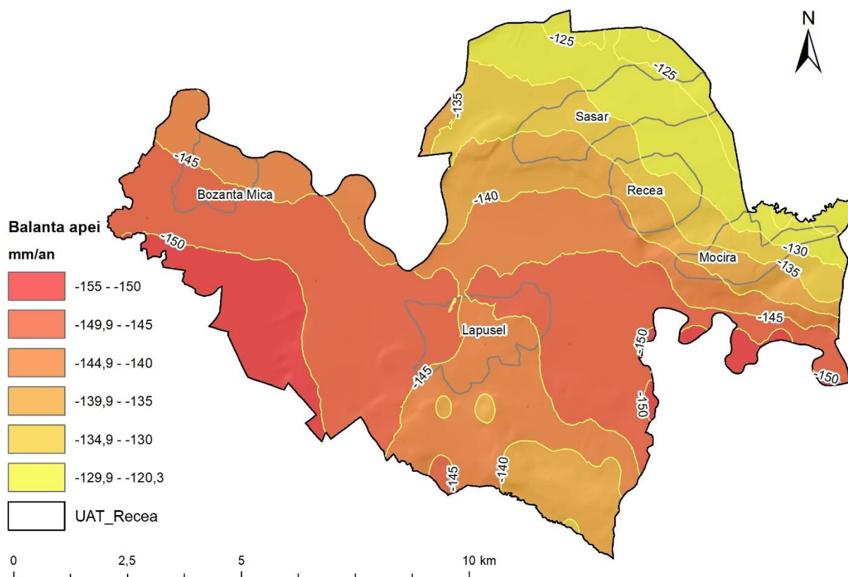
Fig. 7 – Distribuția balanței apei în Comuna Recea
