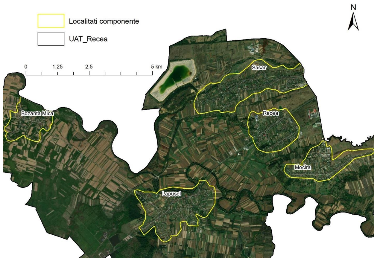
Fig. 11 – Localitățile componente ale comunei Recea
