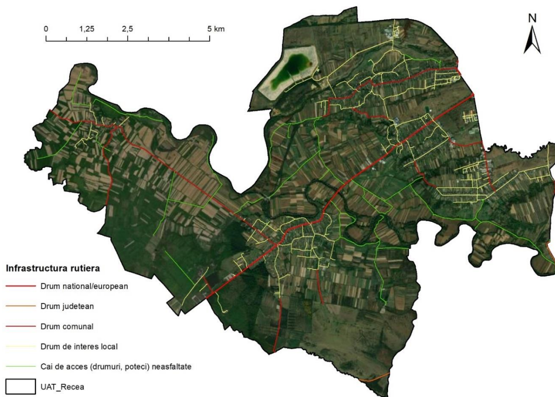
Fig. 14 – Harta infrastructurii rutiere in perimetrul comunei Recea
