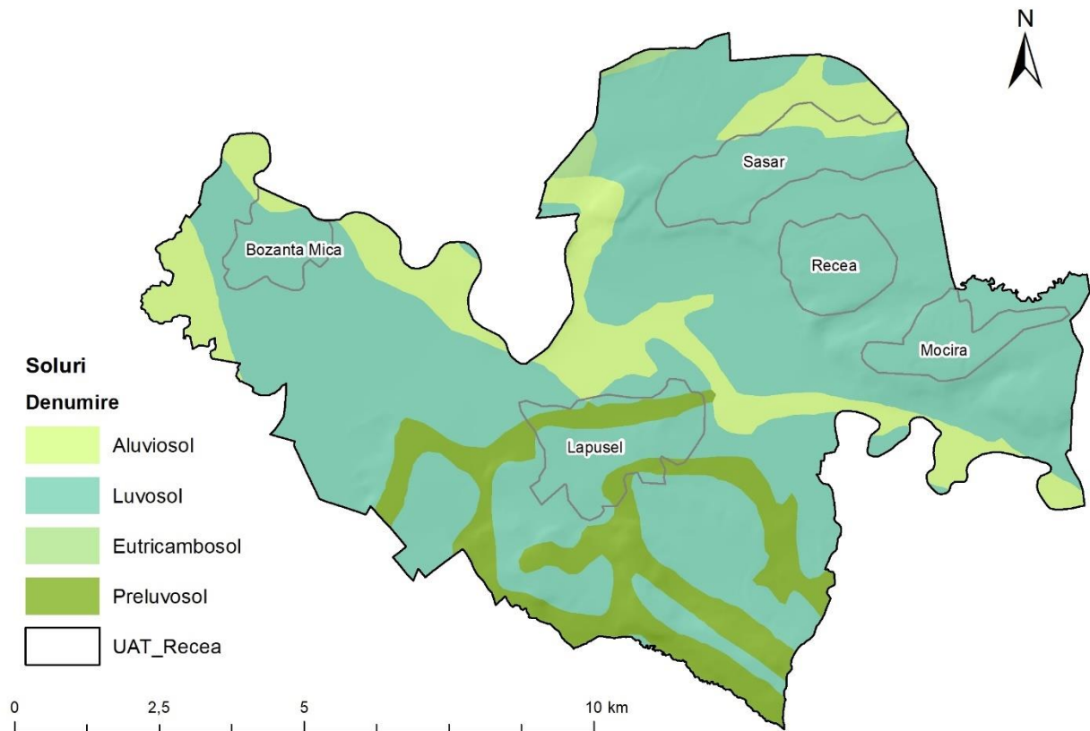
Fig. 9 – Distribuția solurilor în Comuna Recea
