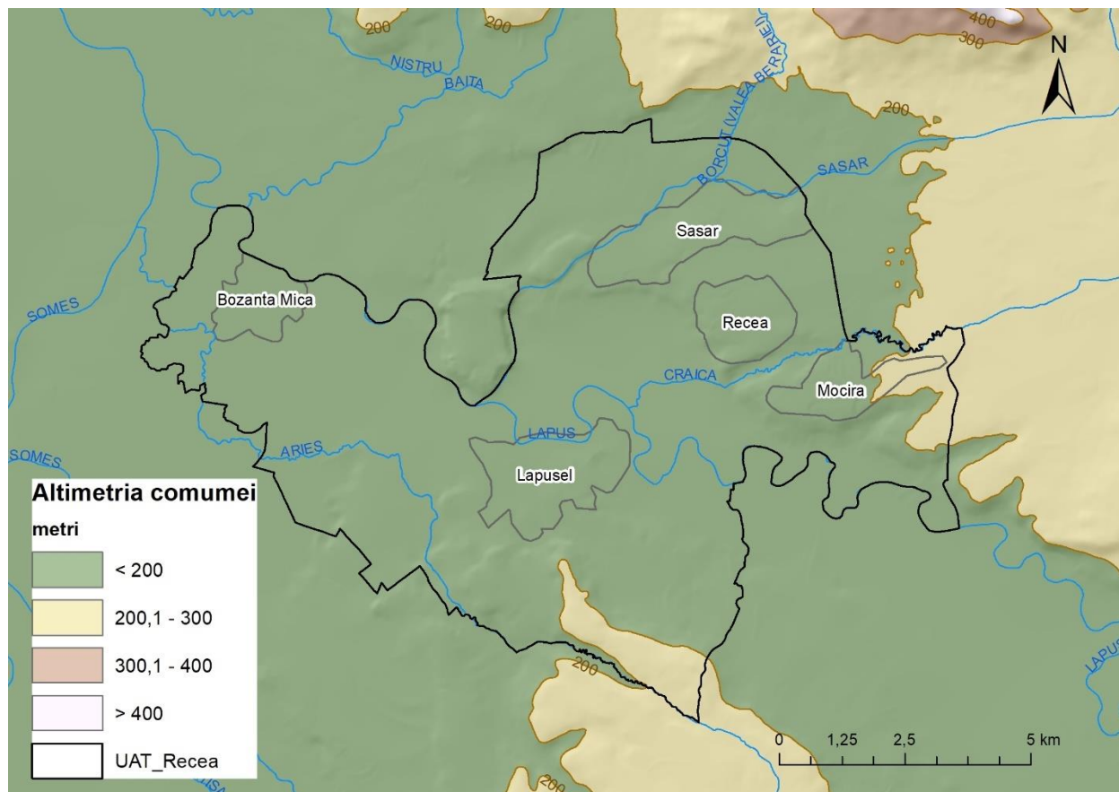
Fig. 3 – Harta altimetrică a comunei Recea
