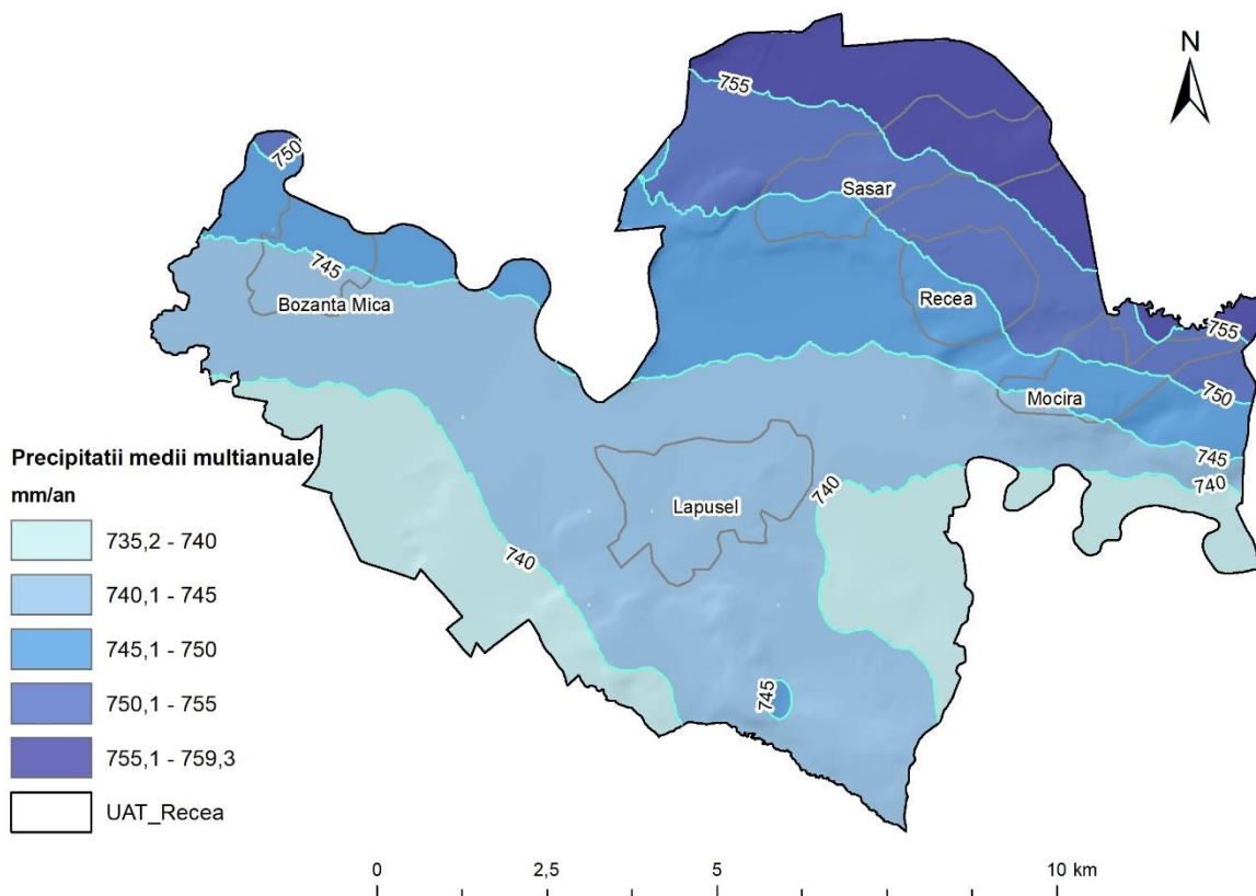
Fig. 5 – Distribuția precipitațiilor în Comuna Recea
