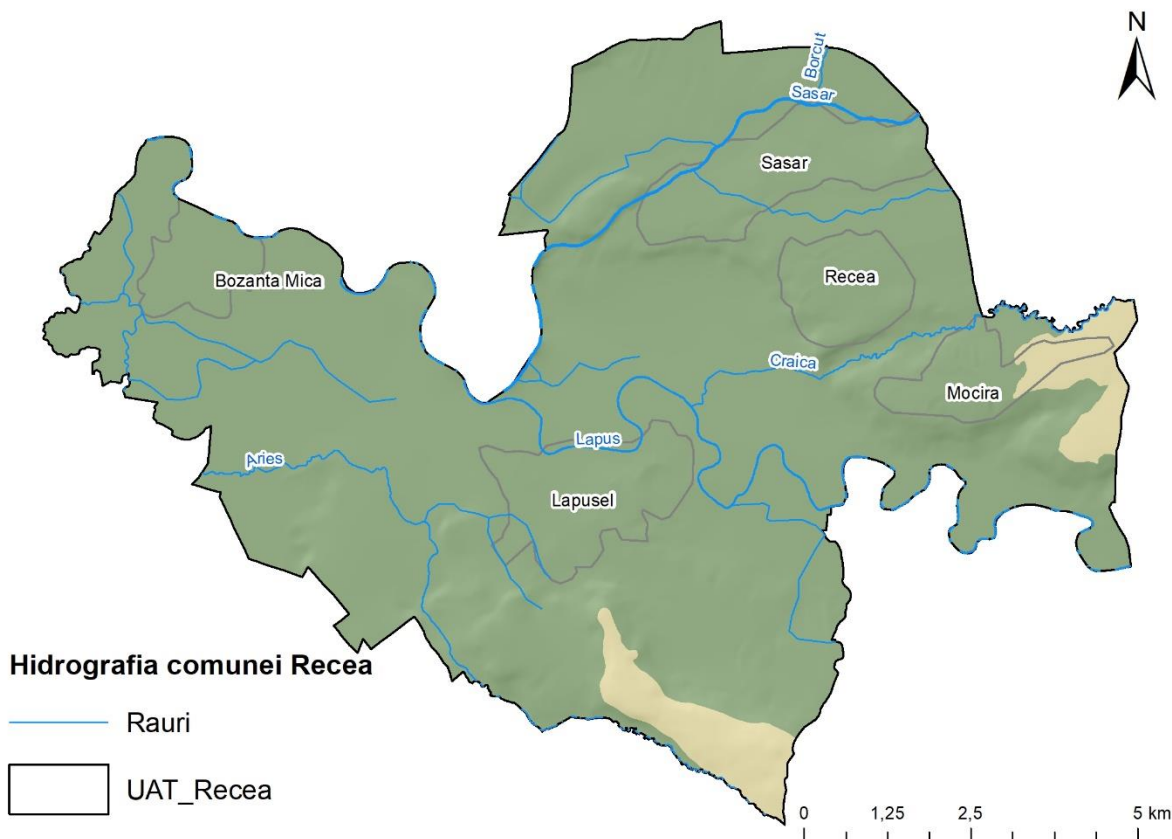
Fig. 8 – Distribuția râurilor în Comuna Recea
