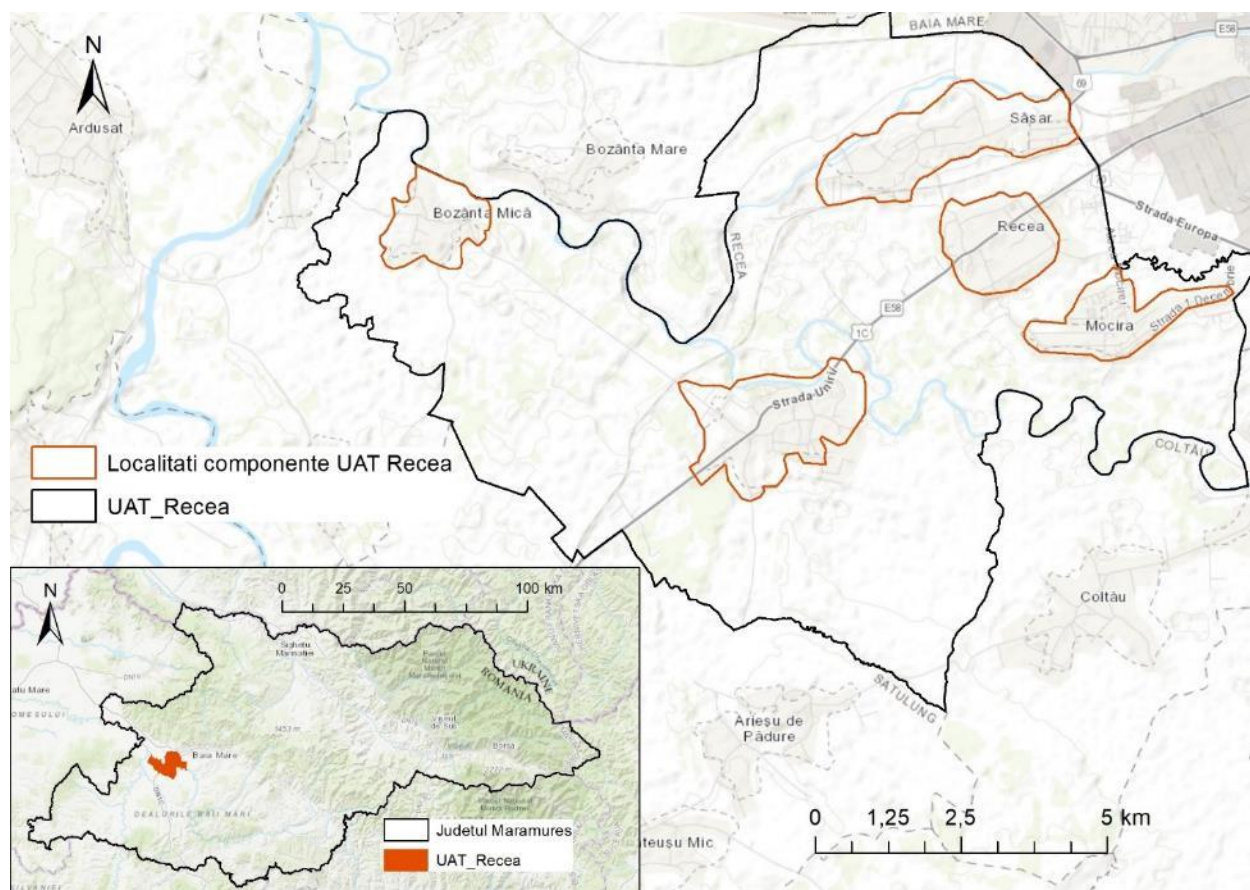
Fig. 1 – Localizarea comunei în perimetrul județului Maramureș
